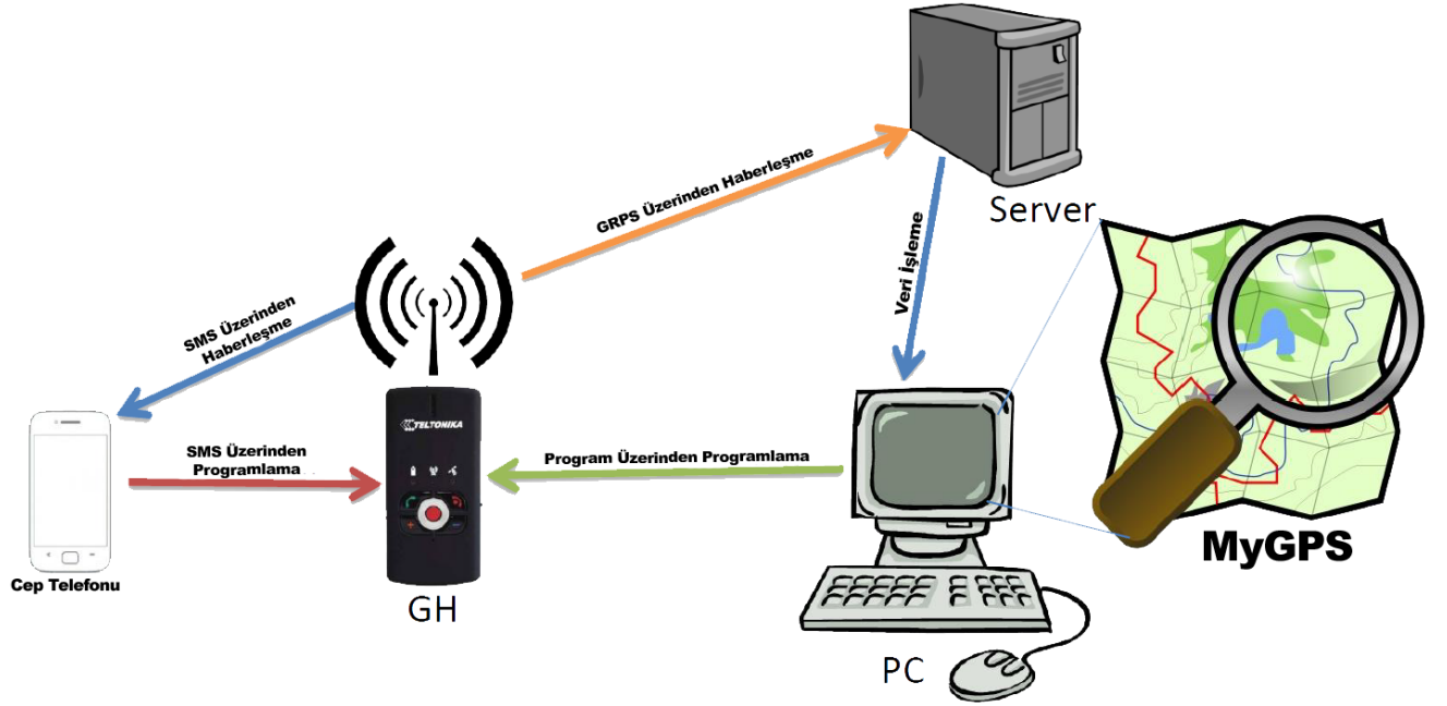
Şekil. 1 Temel GH3000 Sistem Yapısı
