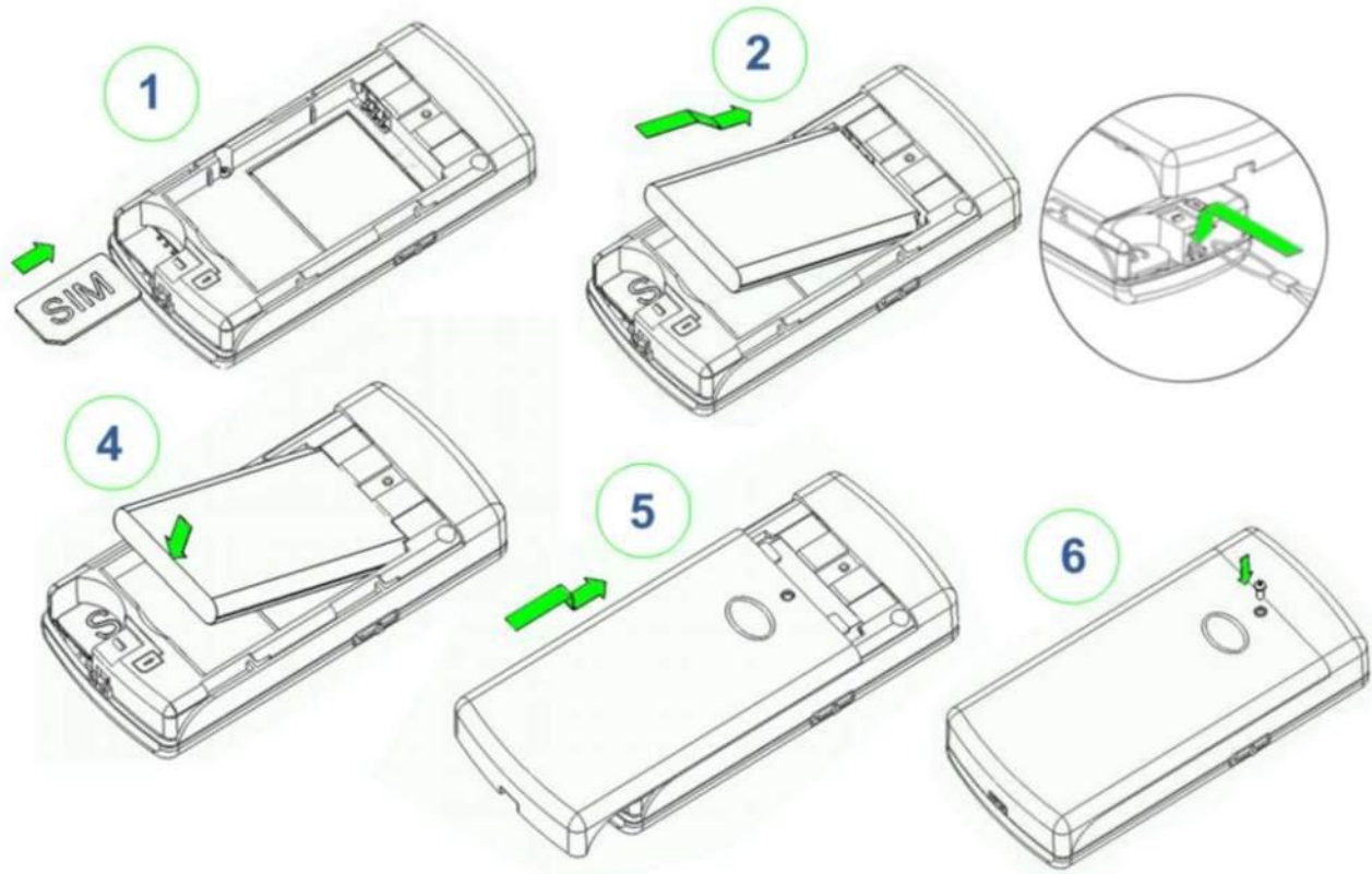
Şekil. 2 GH3000 Çalıştırmaya Hazırlanışı
